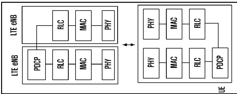
3C type LTE-LTE Interworking : 1f-01 LTE (MeNB), LTE (SeNB)
