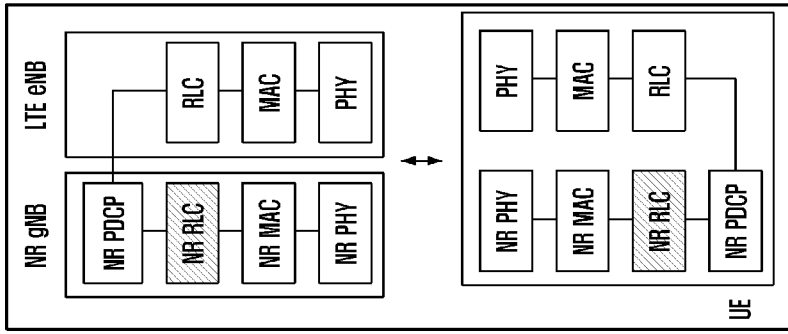
3C type LTE-NR Interworking : 1f-03 NR (MeNB), LTE (SeNB)
