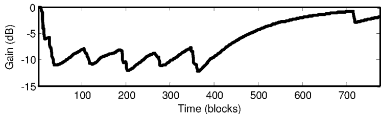
FIG. 10b b) DRC gain
