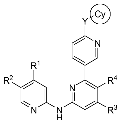
Ic
