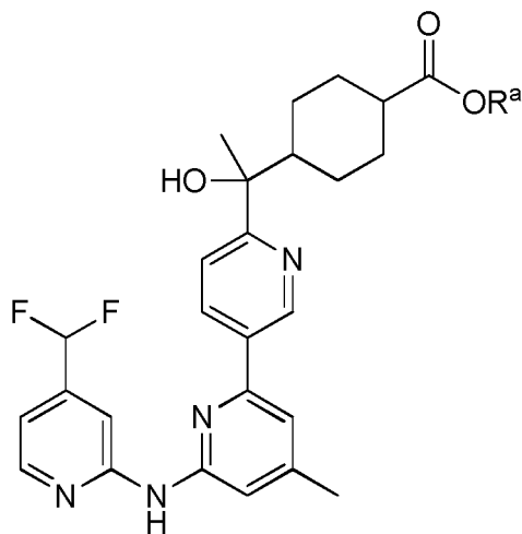
Id
