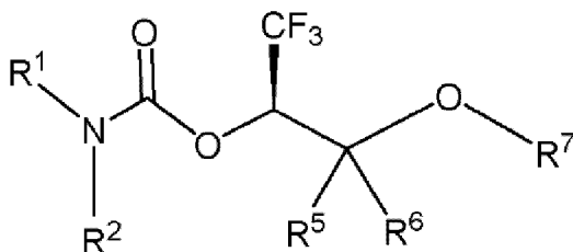
I-a1
