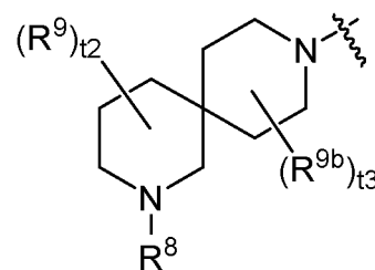
a-46-3
