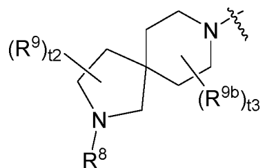
a-46-7
