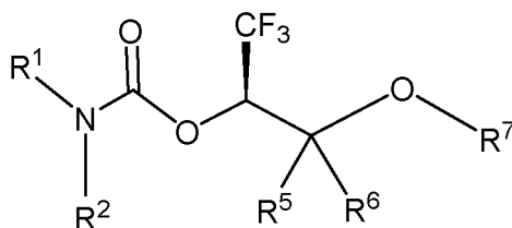
I-a1
