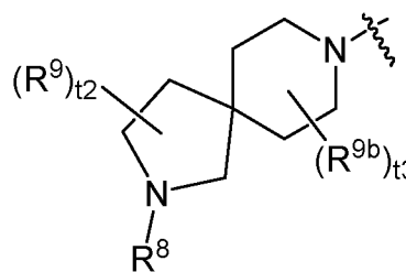
a-46-7
