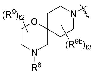
a-46-1
