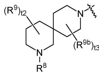
a-46-3
