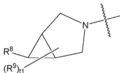
a-13,
