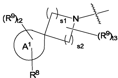
a-6
