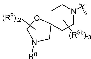
a-46-4
