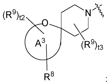
a-36
