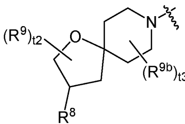
a-46-2
