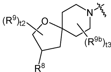
a-46-2
