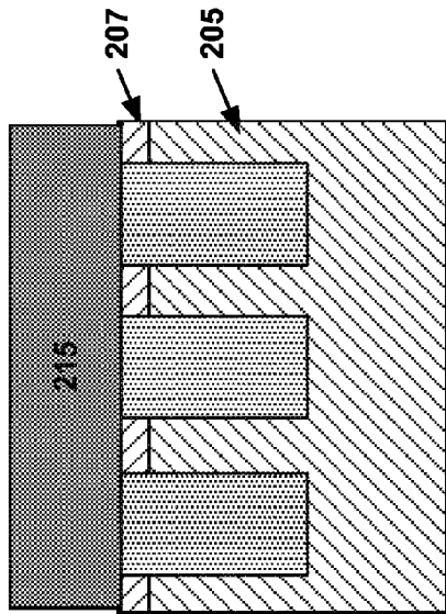
SECTION YY1-YY1 FIG. 7B
