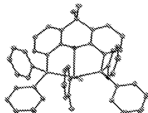
Xantphos (118)
