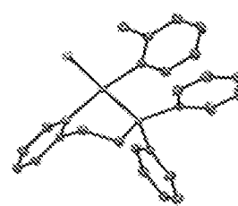
pyphos (119)
