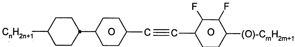
CPTP-n(O)mFF
