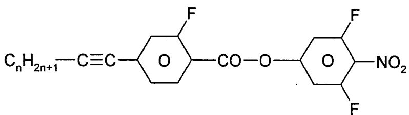
GZU-nA-NO2
