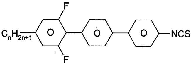
UPP-n-S
