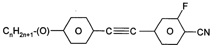
PTG-n(O)-N
