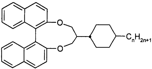
B(OC)2C*H-C-n
