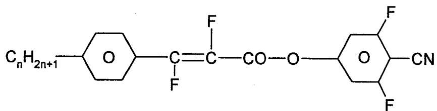
PWZU-3-N
