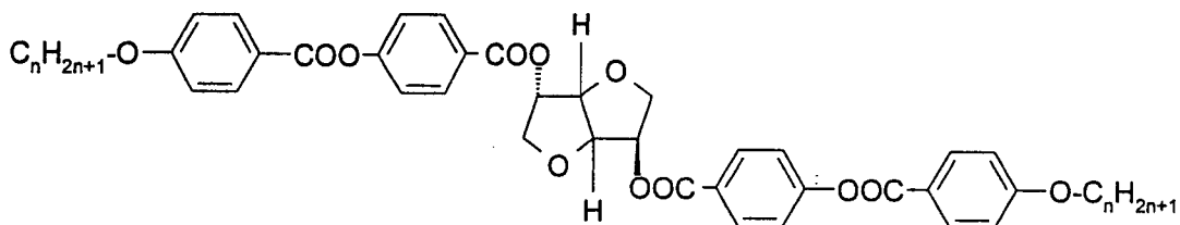
(n0PZPZ)2X*
