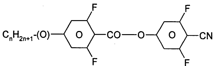
UZU-n(O)-N
