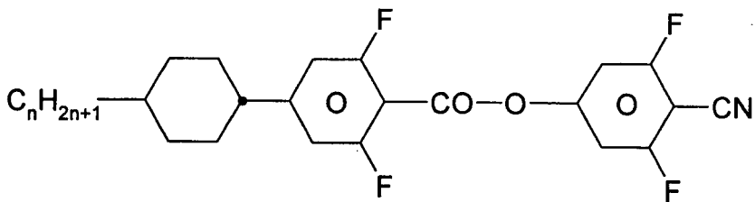
CUZU-n-N
