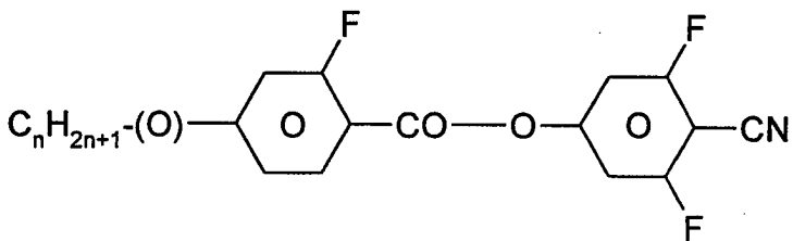
GZU-n(O)-N
