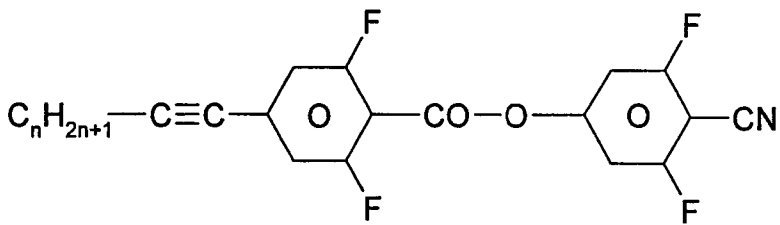
UZU-nA-N
