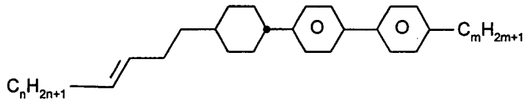
CPP-nV2-m
