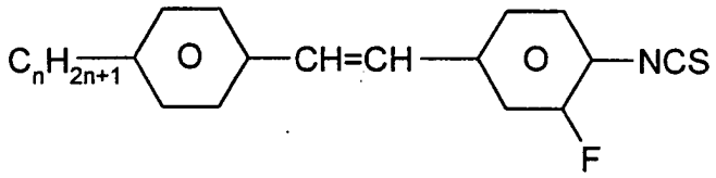
PVG-n-S
