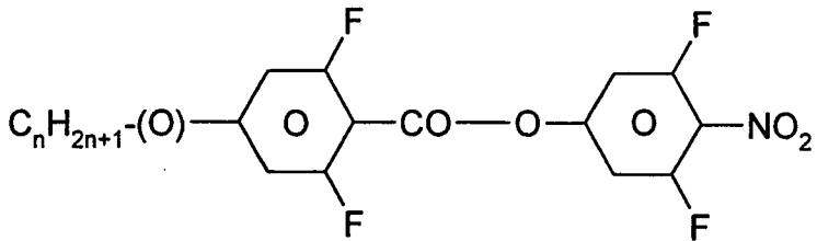
UZU-n(O)-NO2
