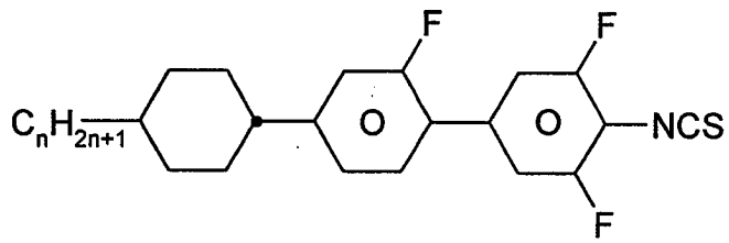
CGU-n-S
