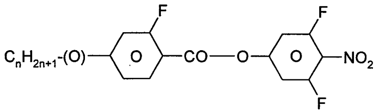
GZU-n(O)-NO2
