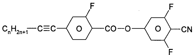
GZU-nA-N
