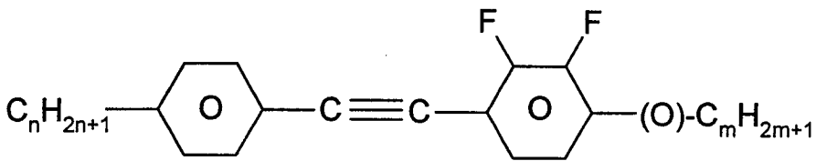
PTP-n(O)mFF
