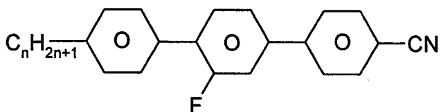
PGIP-n-N
