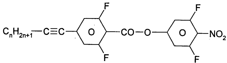
UZU-nA-NO2
