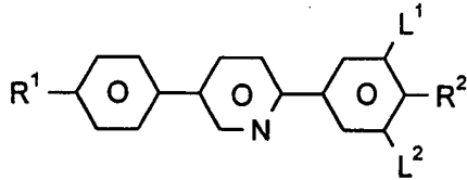
PPYRP
