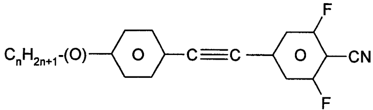
PTU-n(O)-N
