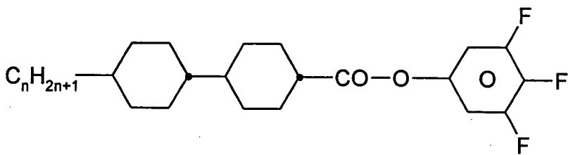
CCZU-n-F
