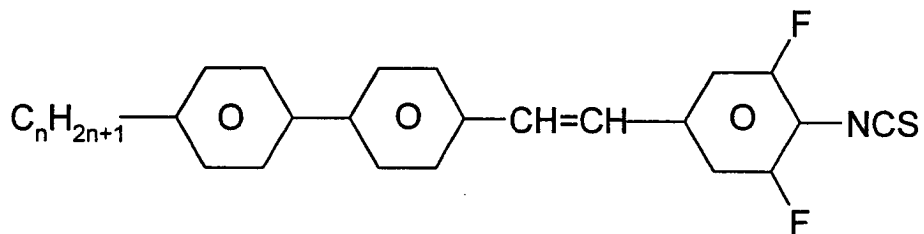
PPVU-n-S
