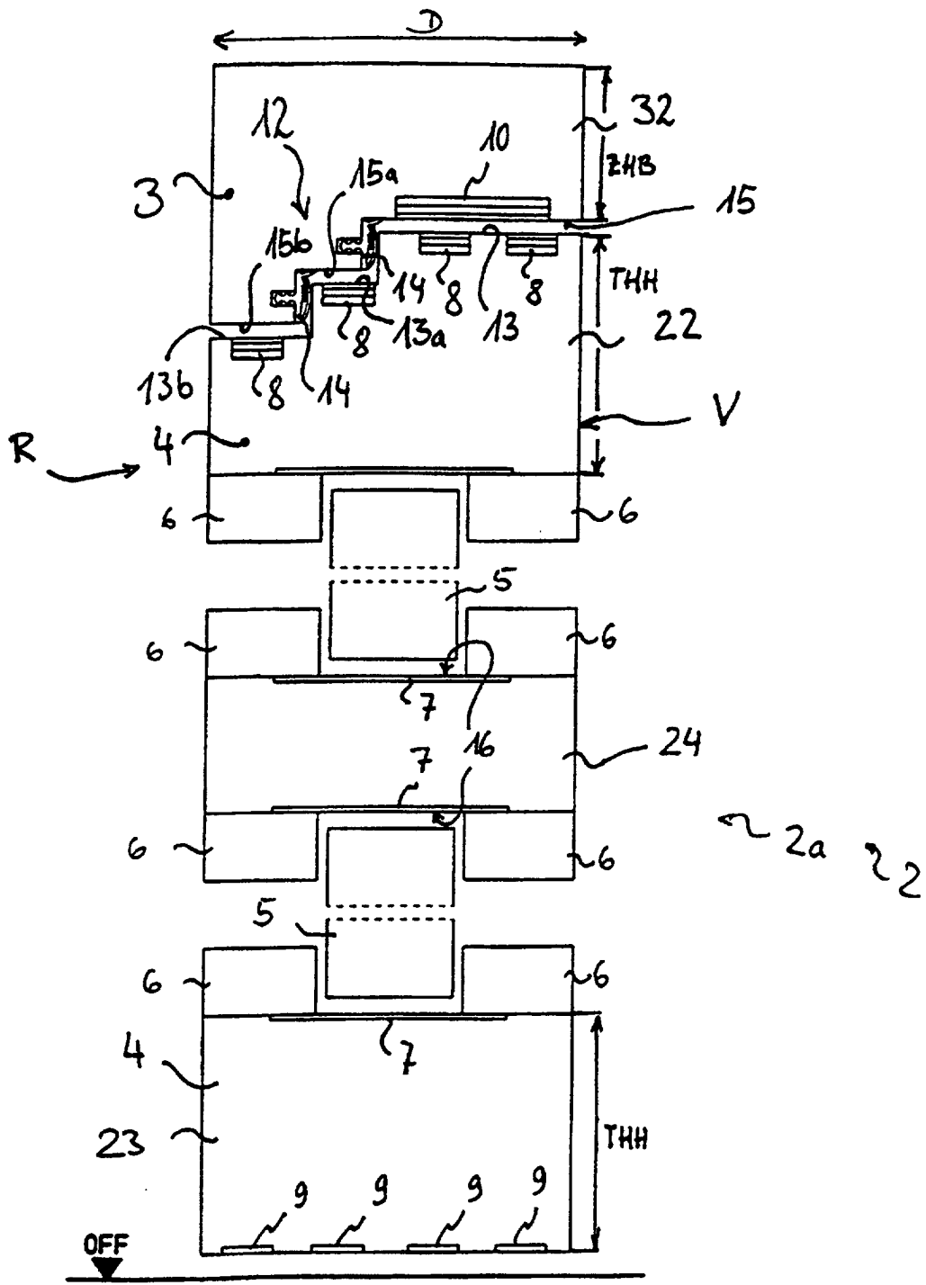
▲ Vertikalschnitt A2 - A2
