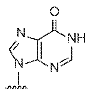
inosine
