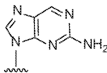
2-aminopurine
