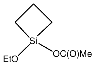
1-ethoxy-1-acetoxy-1-silacyclobutane
