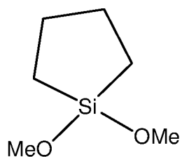
1,1-dimethoxy-1-silacyclopentane
