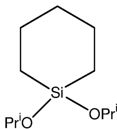
1,1-di-iso-propoxy-1-silacyclohexane
