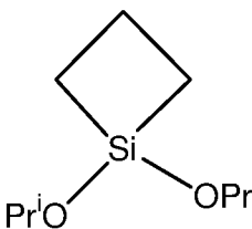
1,1-di-isopropoxy-1-silacyclobutane
