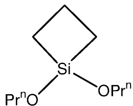
1,1-di-n-propoxy-1-silacyclobutane
