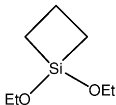
1,1-diethoxy-1-silacyclobutane
