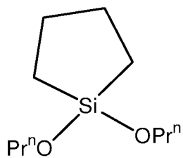
1,1-di-n-propoxy-1-silacyclopentane
