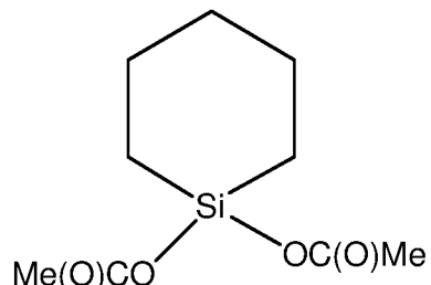
1,1-diacetoxy-1-silacyclohexane
