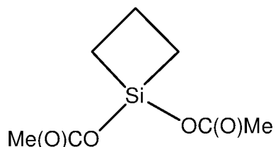
1,1-diacetoxy-1-silacyclobutane
