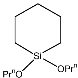
1,1-di-n-propoxy-1-silacyclohexane
