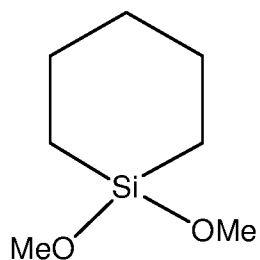
1,1-dimethoxy-1-silacyclohexane
