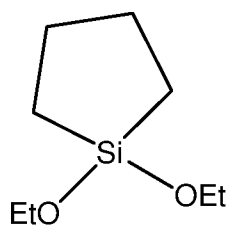
1,1-diethoxy-1-silacyclopentane
