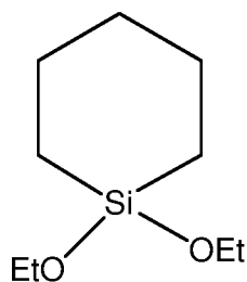
1,1-diethoxy-1-silacyclohexane
