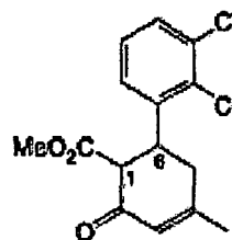
Substance 25 (1,6 trans)
