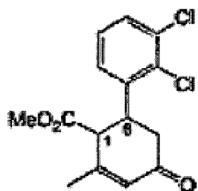
Substanz 23 (1,6 cis)
