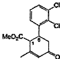
Substance 23 (1,6 cis)
