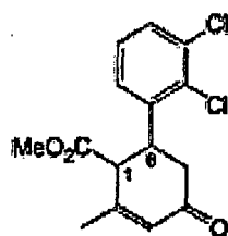
Substance 23 (1,6 cis) Substance 24 (1,6 trans)
