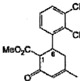
Substanz 25 (1,6 trans)
