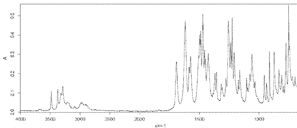
Polymorph IV
