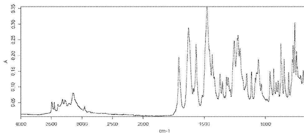
Polymorph V
