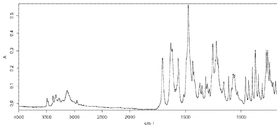
Polymorph I
