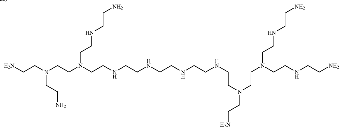
Polyethylenimine (PEI)
