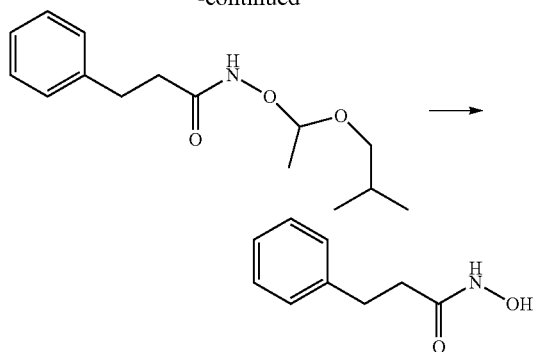
N-(1-isobutoxyethoxy)-3-phenylpropionamide
