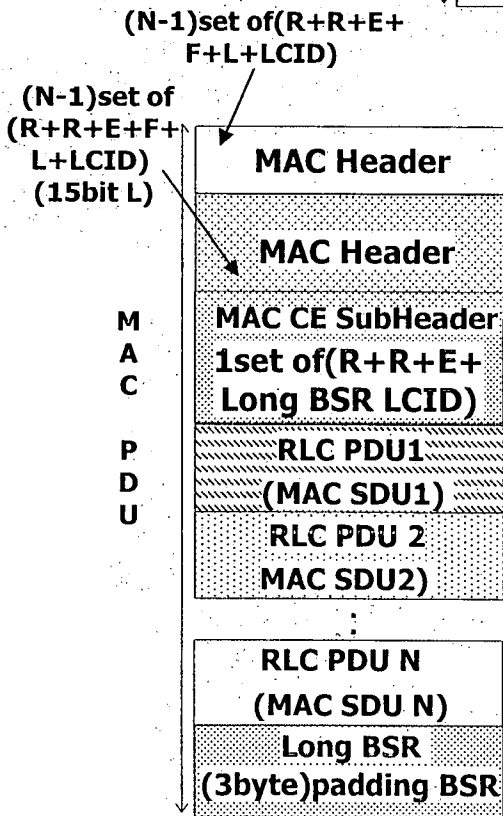
(b) case 2, explicit padding BSR
