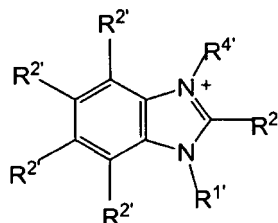
Benzimidazolium
