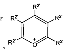
Pyrilium
