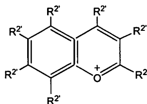
Chromylium (1-Benzopyrylium)
