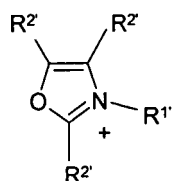
Oxazolium
