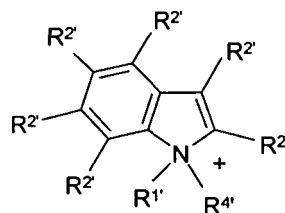
Indolium
