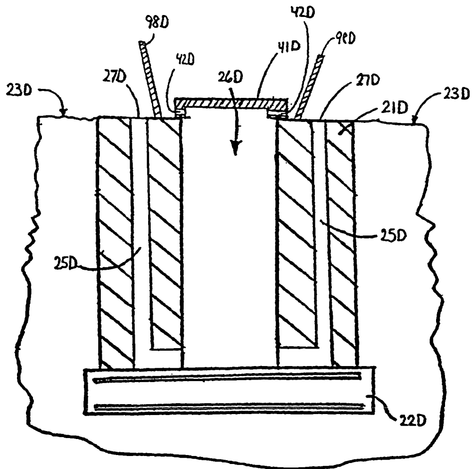
FIG. 8D
