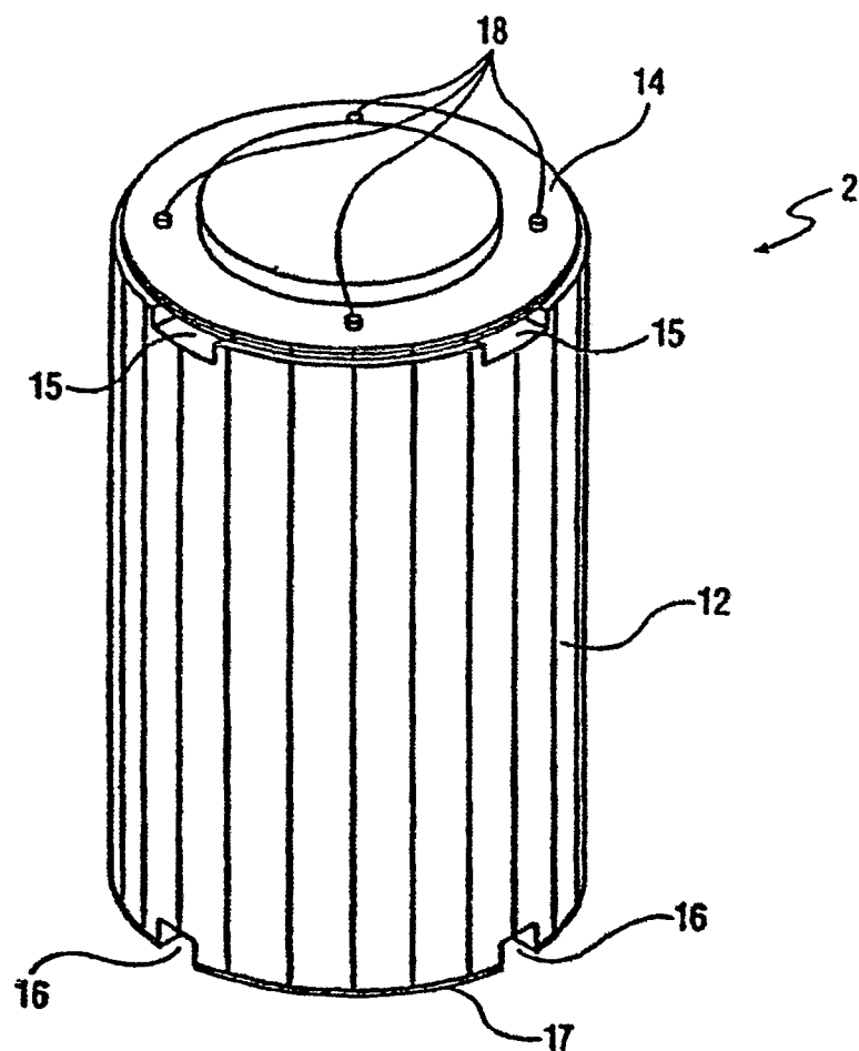
FIG. 1 TÉCNICA ANTERIOR
