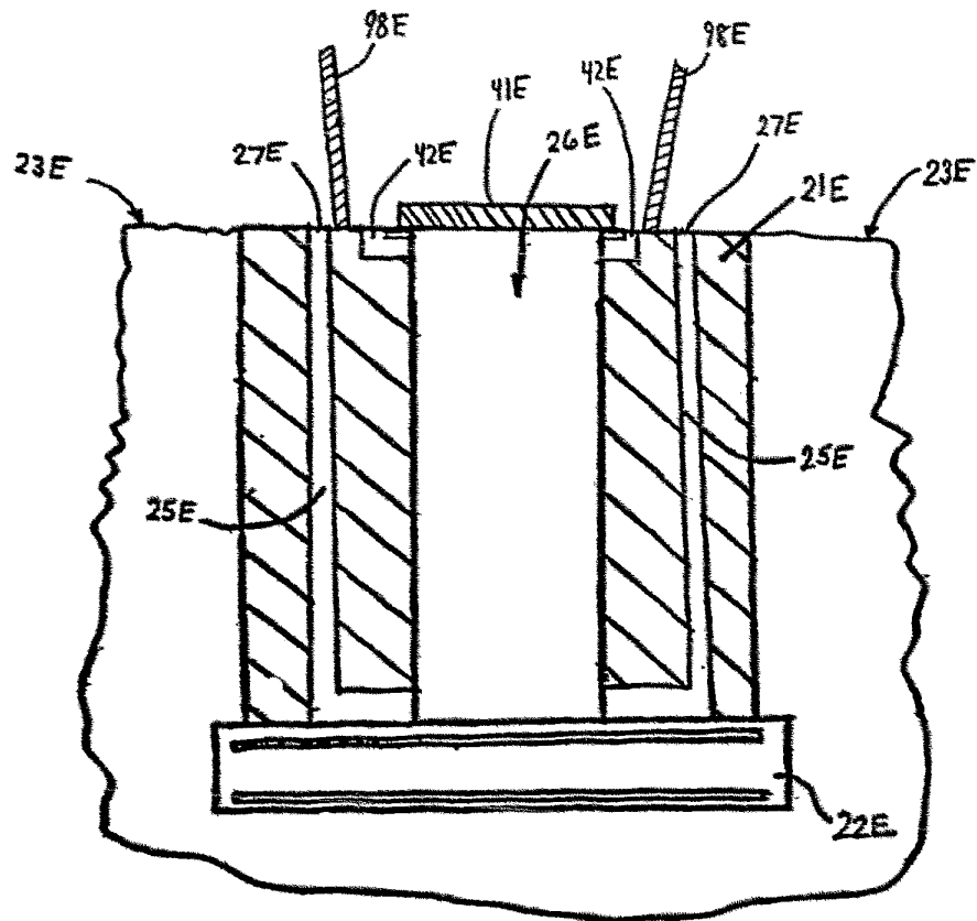
FIG. 8E
