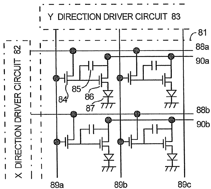
FIG. 24A EL PANEL CIRCUIT DIAGRAM
