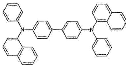
( \alpha -NPD)
