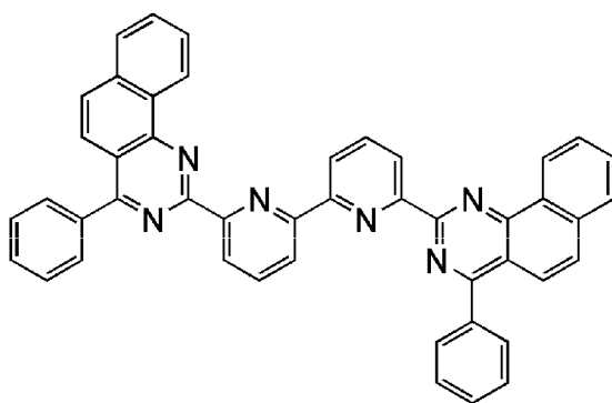
(401) 6,6'(P-Bqn)2BPy
