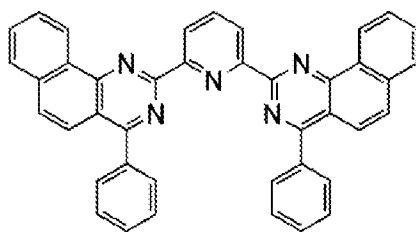
(100) 2,6(P-Bqn)2Py
