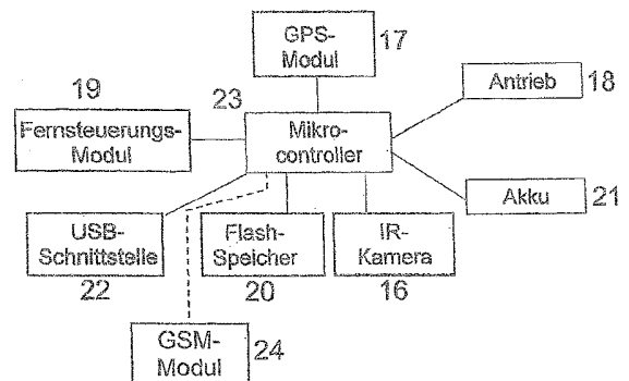
Kleinfluggerät
