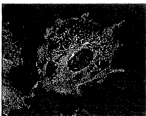
AAG 7 500nM
