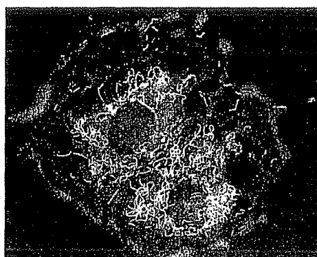
AAG 1 250nM
