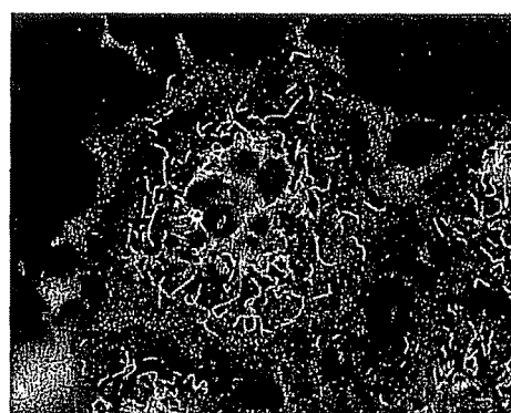
AAG 16 40nM
