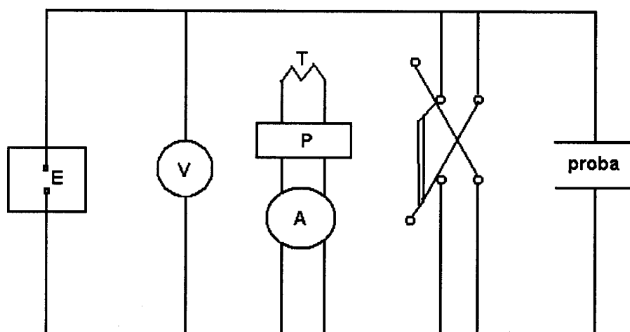
Schema instalației pentru studiul proprietăților electrice ale compuşilor revendicați E – sursă de curent; V - voltmetru electronic; A – miliampermetru pentru intensități mici; P – potențiometru; T – termocuplu.
