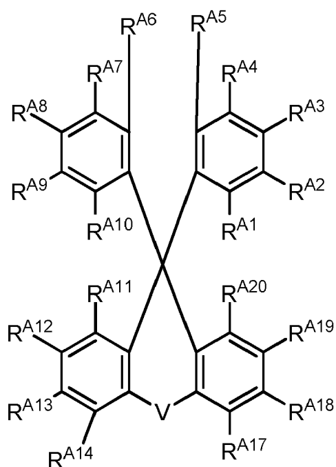
Formula IIg.
