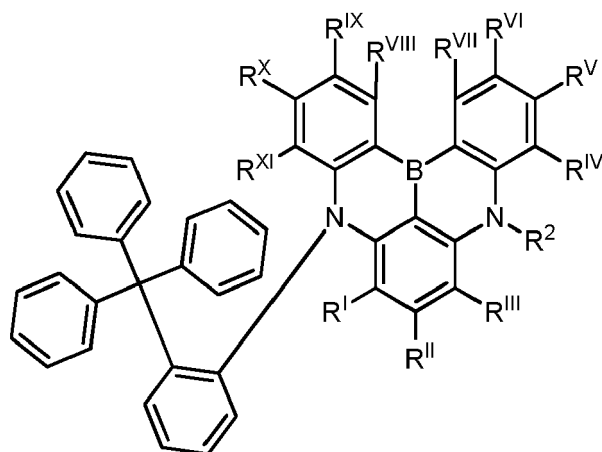
Formula Va
