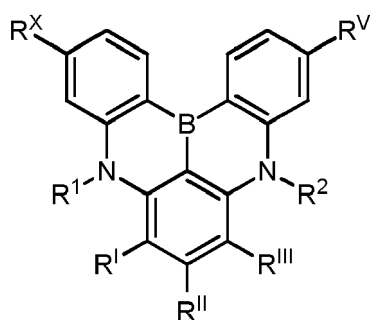
Formula Ic
