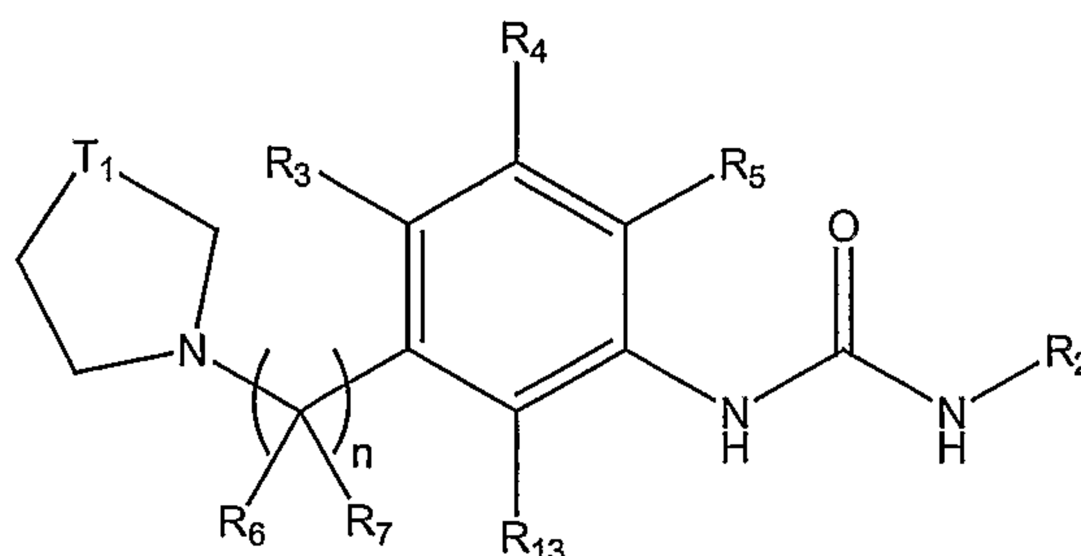
Formula Ic
