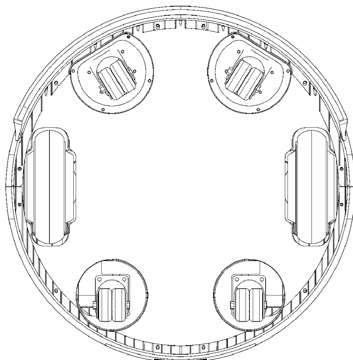
【仰視圖】
