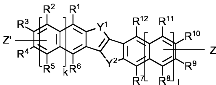
Structure A'
