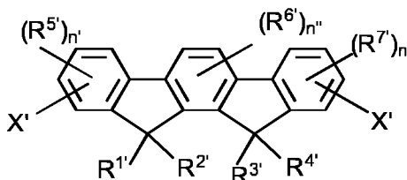
Structure A'
