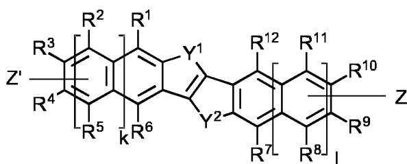
Structure A'
