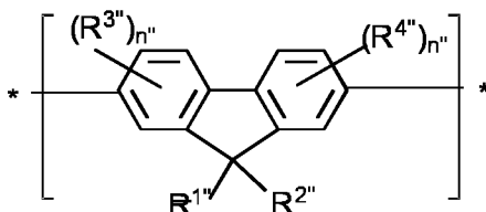
(Q)
