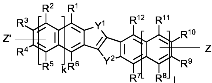
Structure A'
