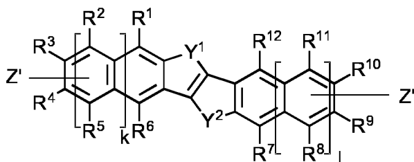
Structure A'
