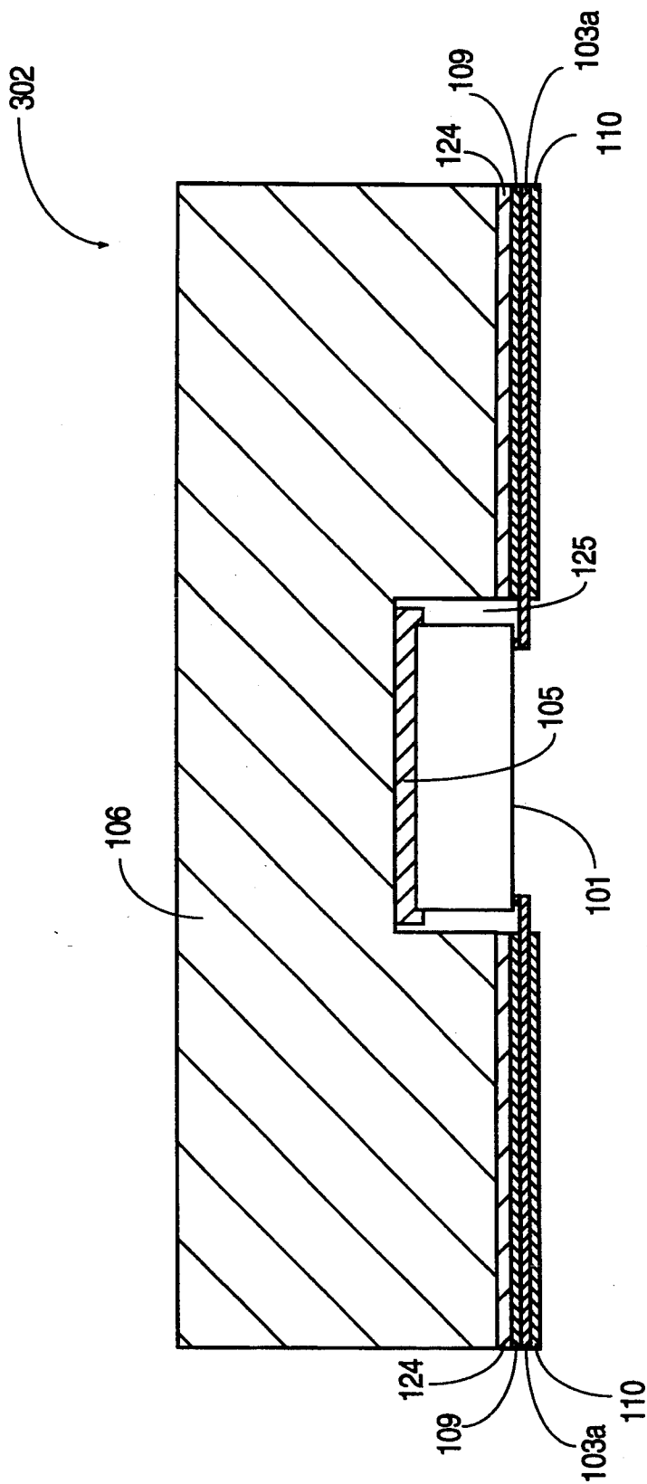
DIE ATTACH
