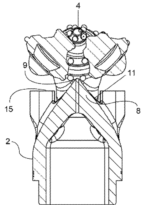
SECTION D-D
