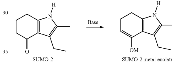
SUMO-2
