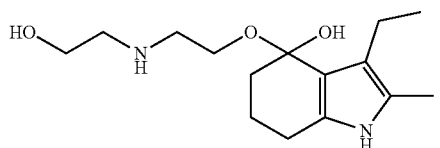
SUMO-3 isomer
