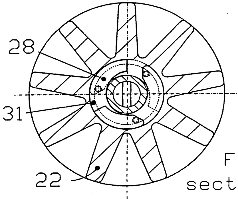
Fig. 4D section A-A
