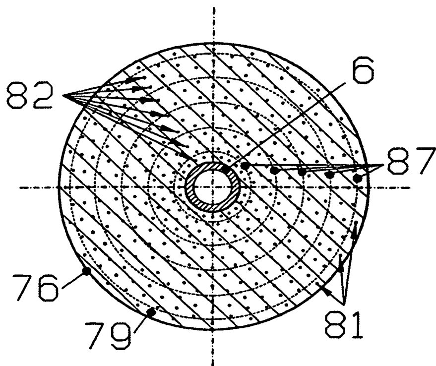
Fig. 7D section E-E
