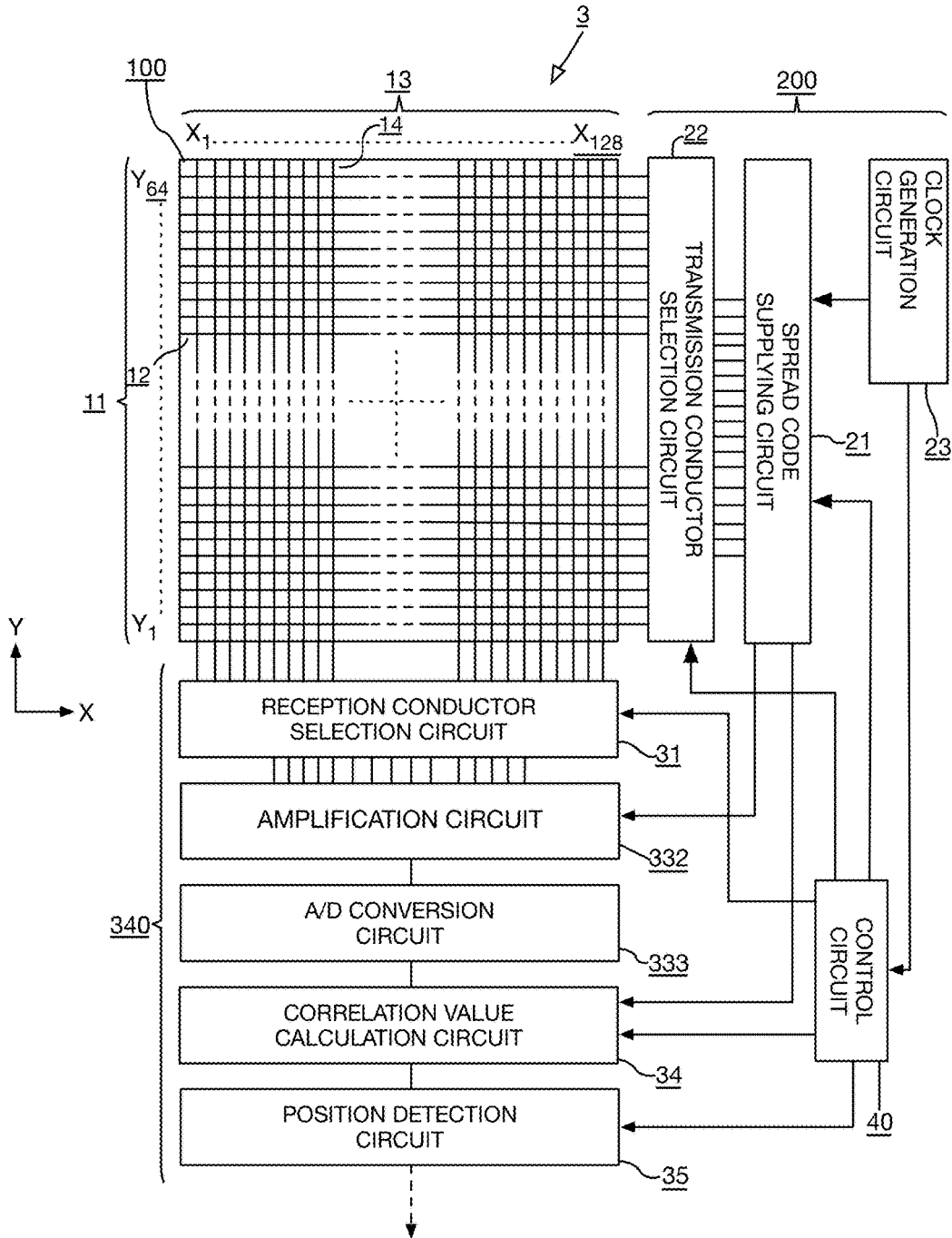
FIG. 23 (PriorArt)
