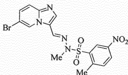
Imidazo[1,2-a]pyridine
