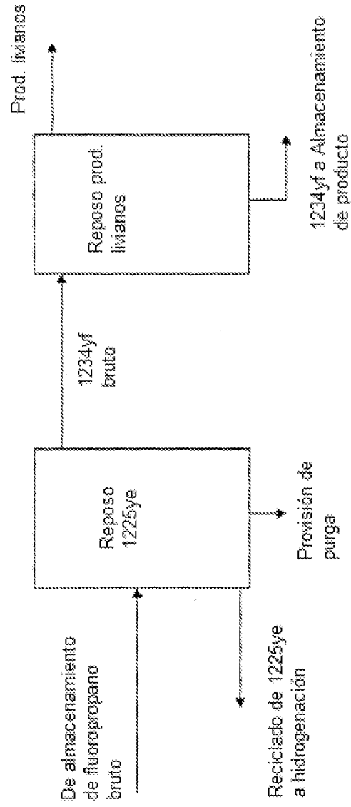
Figura 3: Purificación de 1225yf y 1234yf
