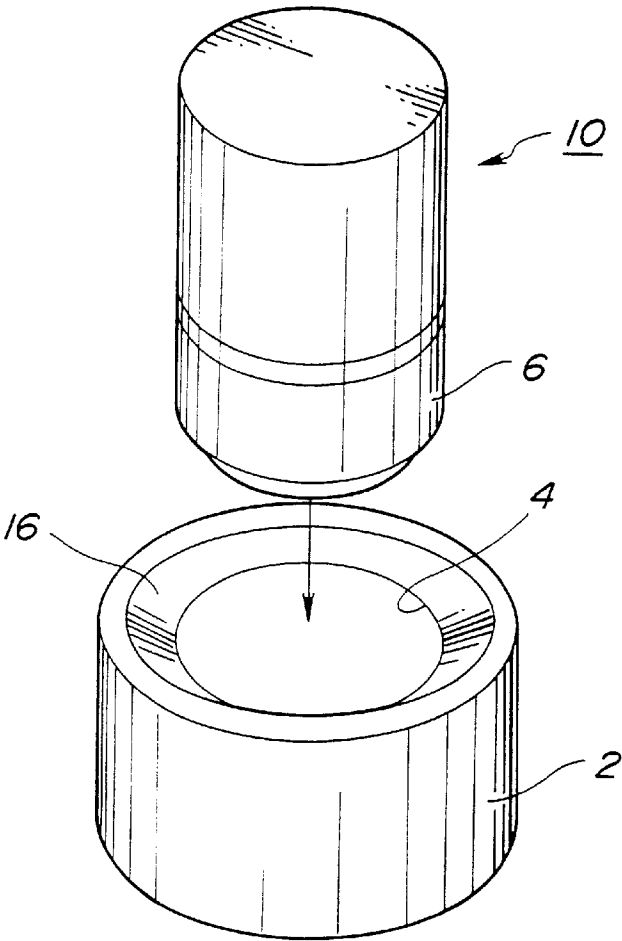
FIG. 3B
