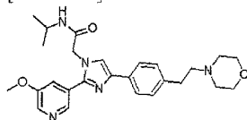
[Chem. 265]
