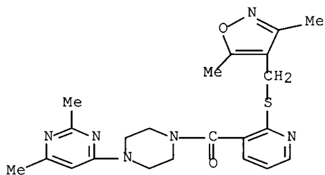
[4-(5-bromo-2-pyrimidinyl)-1-piperazinyl][2-[(5-methyl-3-isoxazolyl)methyl]thio]-3-pyridinyl]-methanone
