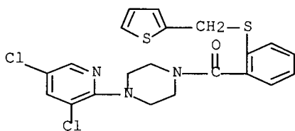
[4-(3,5-dichloro-2-pyridinyl)-1-piperazinyl][2-[[[(2-thienylmethyl)thio]phenyl]-methanone
