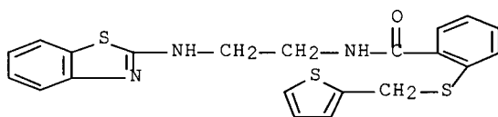
N-[2-[(3-cyano-2-pyridinyl)amino]ethyl]-2-[(4-thiazolylmethyl)thio]-benzamide
