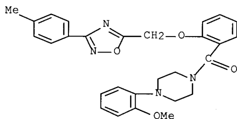
[2-[(3,5-dimethyl-4-isoxazolyl)methoxy]phenyl][4-(2-methoxyphenyl)-1-piperazinyl]-
