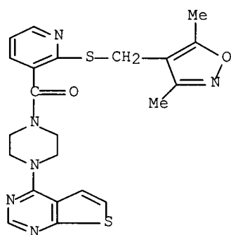
[2-[[[(3,5-dimethyl-4-isoxazolyl)methyl]thio]-3-pyridinyl][4-(3-methoxyphenyl)-1-piperazinyl]-methanone
