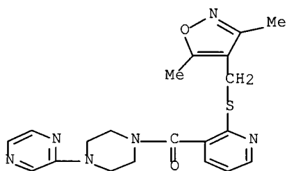
[2-[[[(5-methyl-3-isoxazolyl)methyl]thio]-3-pyridinyl][4-(2-pyridinyl)-1-piperazinyl]-methanone
