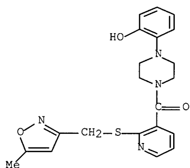
[4-(2-hydroxyphenyl)-1-piperazinyl][2-[[5-methyl-3-isoxazolyl)methyl]thio]-3-pyridinyl]- methanone
