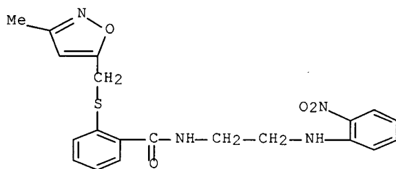
N-[2-[(2-nitrophenyl)amino]ethyl]-2-[(3-thienylmethyl)thio]-benzamide
