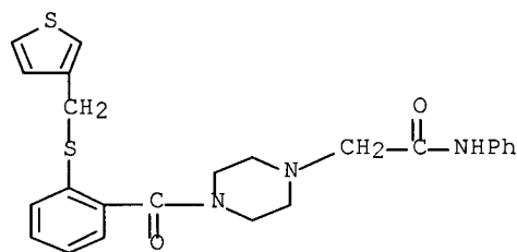
N-(2-chlorophenyl)-4-[[2-[[[(5-methyl-3-isoxazolyl)methyl]thio]-3-pyridinyl]carbonyl]-1-piperazineacetamide
