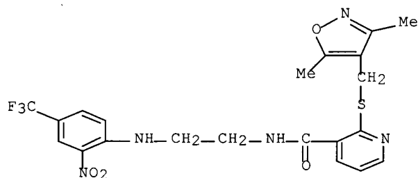
N-[2-((methylphenylamino)propyl)-2-[(4-thiazolylmethyl)thio]- benzamide
