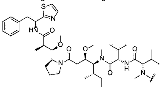
(dolastatin)
