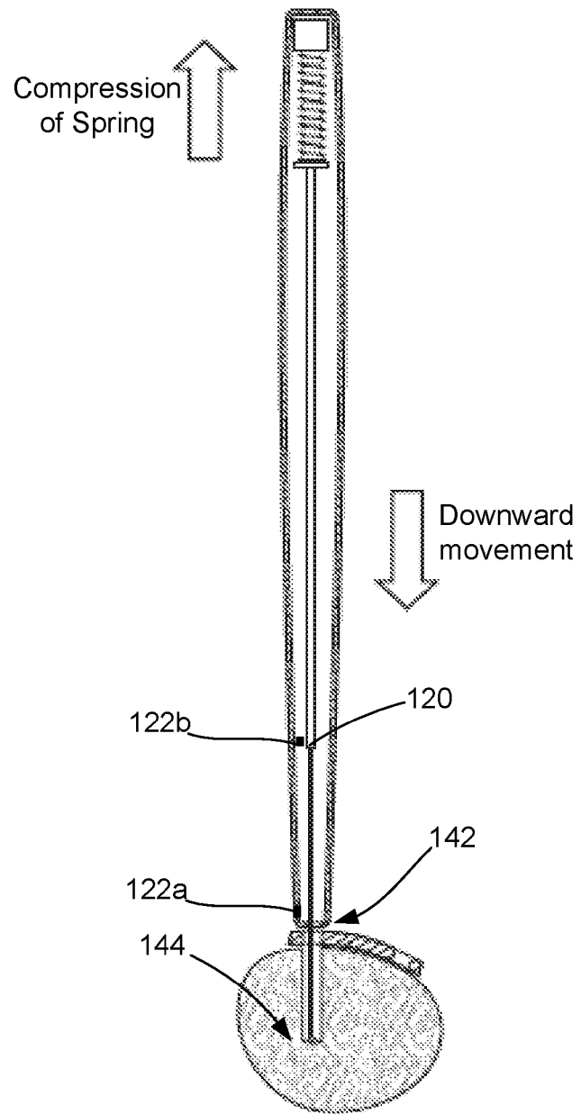
FIG. 4B
