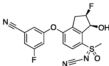
N -(((2 R ,3 S )-7-(3-ciano-5-fluorofenoxi)-2-fluoro-3-hidroxi-2,3-dihidro-1 H -inden-4-il)(metil)(oxo)-λ 6 -sulfanilideno)cianamida ( Compuesto 302 )
