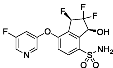
(1 R ,3 S )-1,2,2-trifluoro-7-[(5-fluoro-3-piridil)oxi]-3-hidroxi-indan-4-sulfonamida ( Compuesto 341 )
