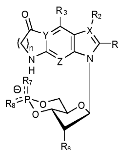
(V)
