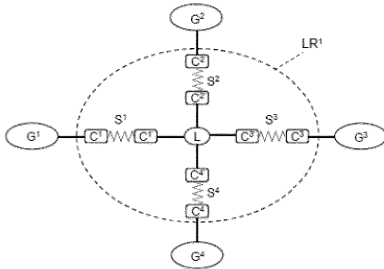
(Ib)
