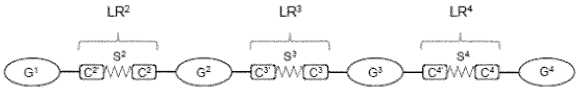
(IIb)
