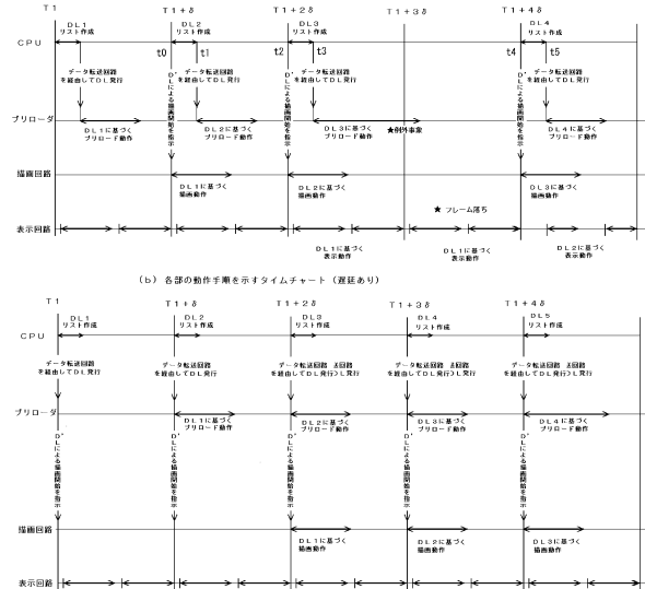
(a) 各部の動作手順を示すタイムチャート(遅延なし)
