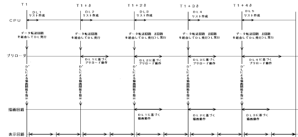
(b) 各部の動作手順を示すタイムチャート（遅延あり）
