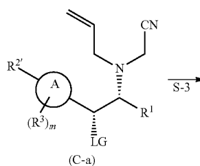
Scheme 3A.
