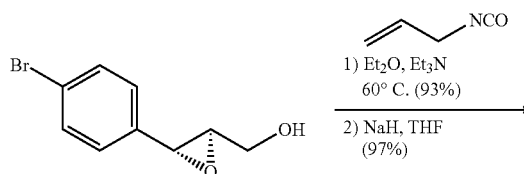
Scheme E1.
