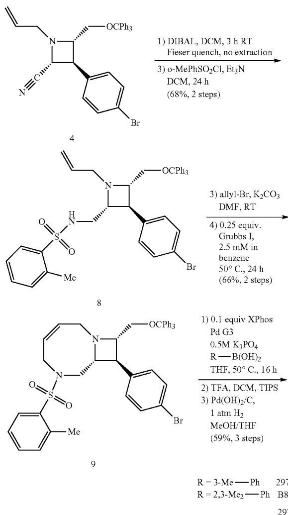
Scheme E3.
