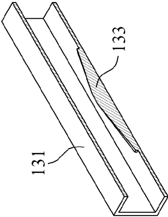
FIG. 5E
