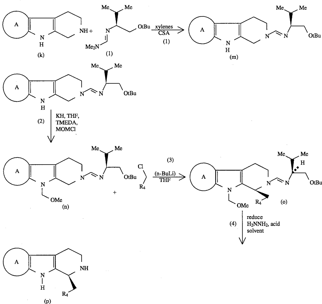
Scheme VI
