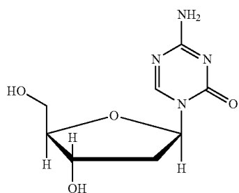
Decitabine
