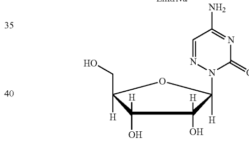
6-Azacitidine
