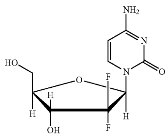
Gemcitabine
