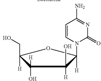
Cytarabine (Ara-C)
