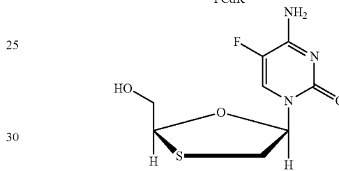
Emtriva
