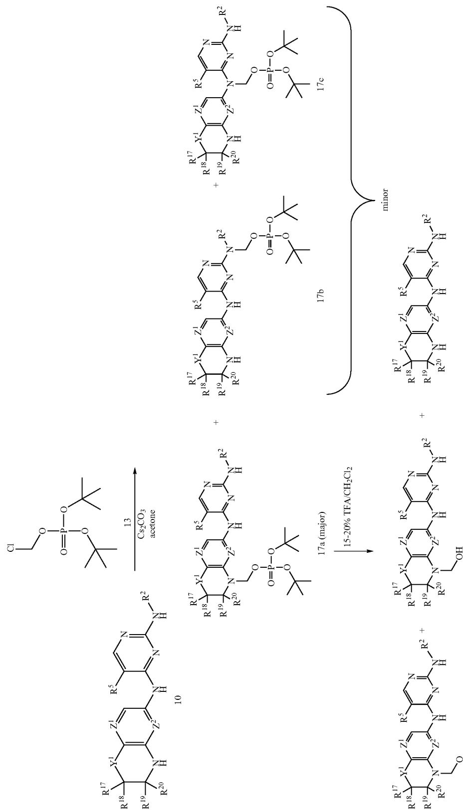
Scheme (IV)
