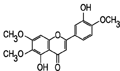
EUPATORIN
