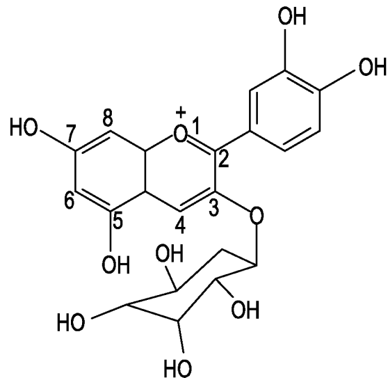
I: CYANIDIN -3- GLUCOSIDE
