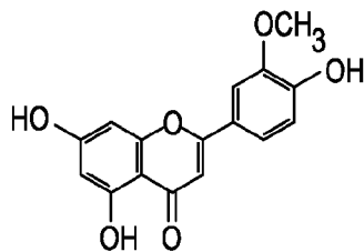
CHRYSOERIOL
