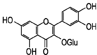
ISOQUERCITRIN
