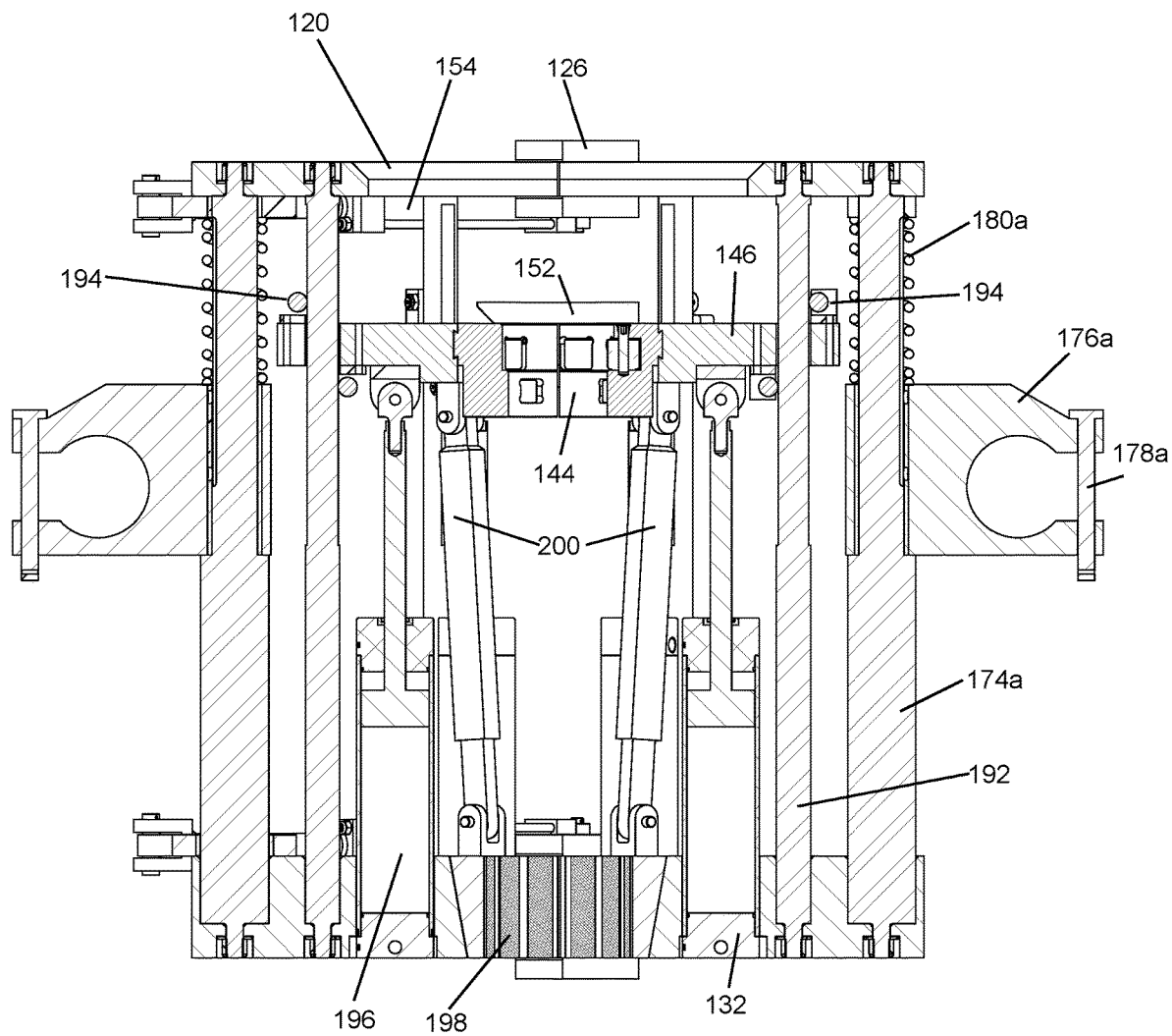
SECTION A-A
