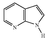
1H-Pyrrolo[2,3-b]pyridine
