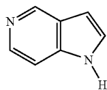
1H-Pyrrolo[3,2-c]pyridine
