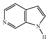
1H-Pyrrolo[2,3-c]pyridine
