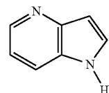
1H-Pyrrolo[3,2-b]pyridine
